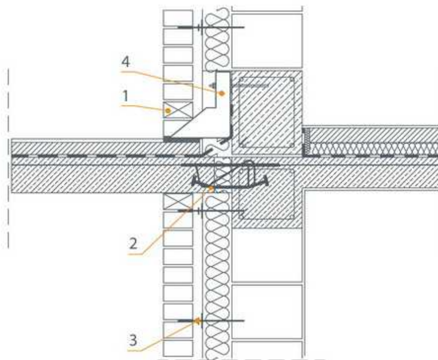
1 - коробка вентиляционная, 2 - балконный термосоединитель 3 - анкер, 4 - кронштейн стальной
