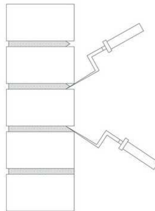
Удаление раствора путем подрезания на глубину 10-15 мм
