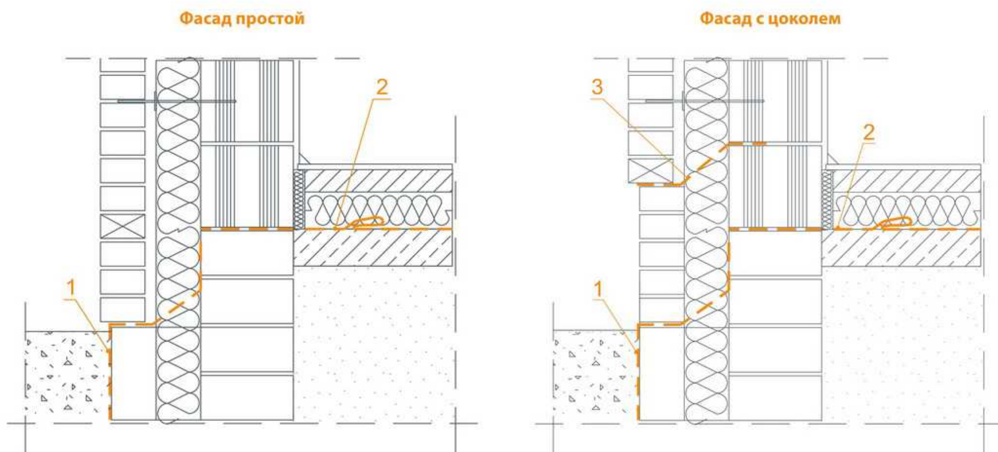
1 - вертикальная изоляция, 2 горизонтальная изоляция, 3 - изоляция цоколь - вентиляционное отверстие
