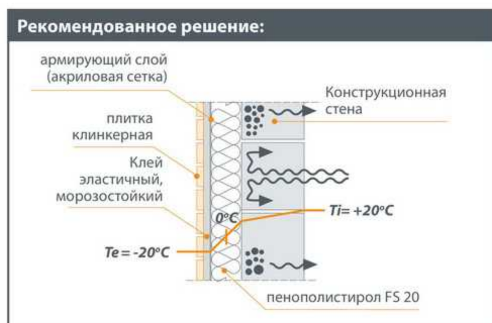
Распределение температур и влажности в стенах утепленных пенополистиролом
