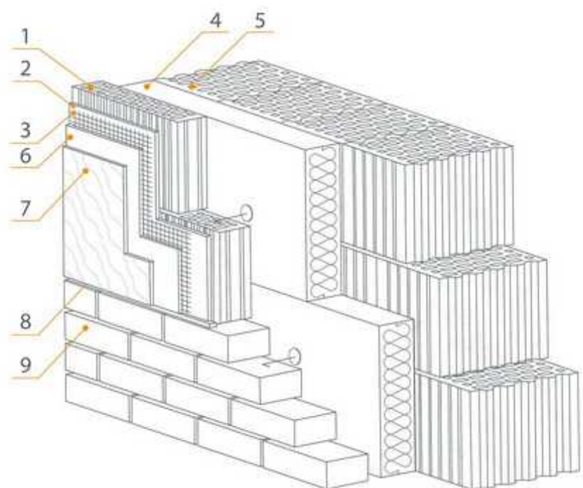
1 - MINI-MAX 88, 2 - цементно-известковая штукатурка, 3 - акриловая сетка, 4 - термоизоляция, 5 - керамический блок, 6 - клей для сетки, 7 - штукатурка, 8 - уплотнительная лента, 9 - клинкерный кирпич
