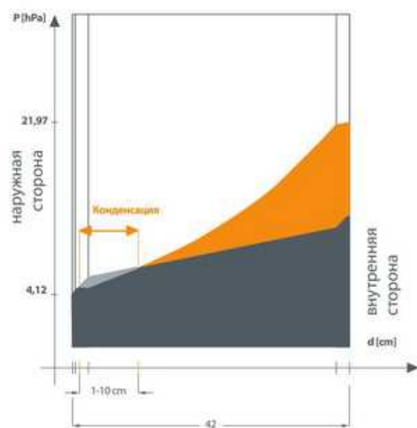
фактическое давление водяного пара в стене
