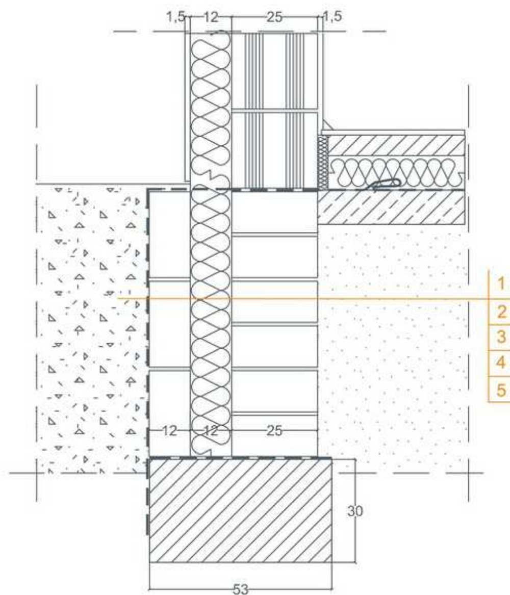
1 пленка, 2 гидроизоляция, 3 блоки бетонные 38x25x12 см 4 теплоизоляция 12 см, 5 блоки бетонные 38x25x12 см
