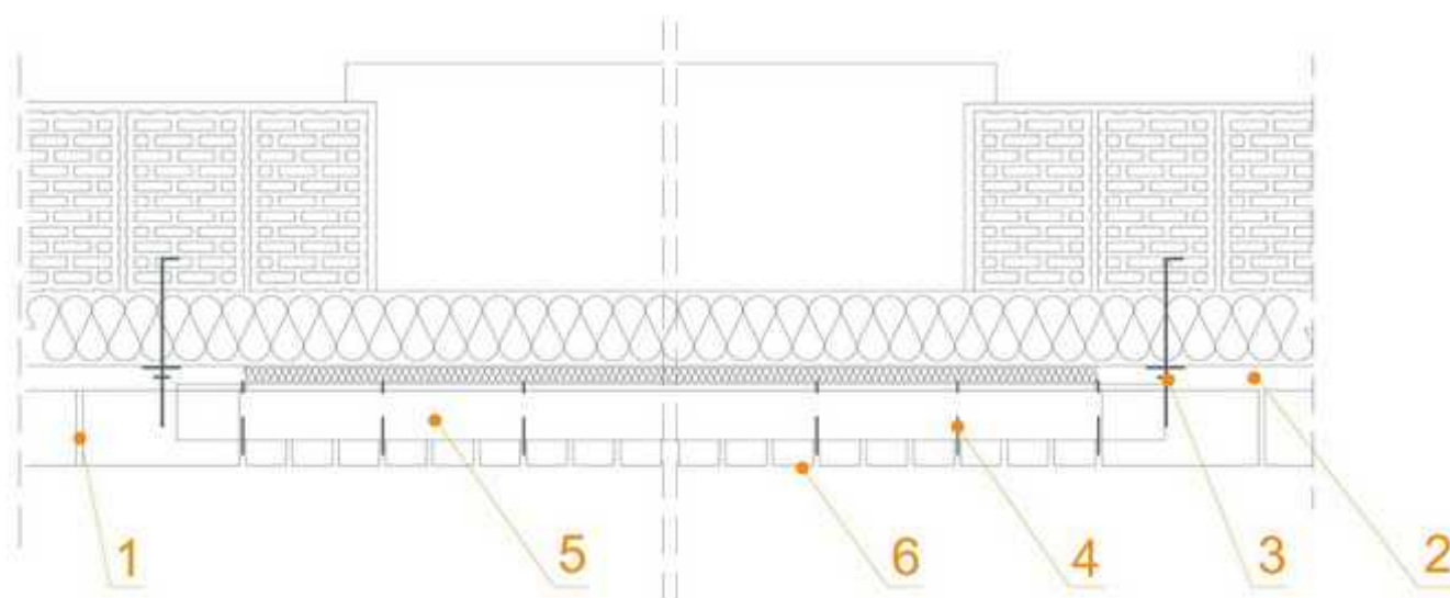
сечение А-А
