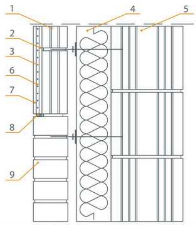
1 - MINI-MAX 88, 2 - цементно-известковая штукатурка, 3 - акриловая сетка, 4 - термоизоляция, 5 - керамический блок, 6 - клей для сетки, 7 - штукатурка, 8 - уплотнительная лента, 9 - клинкерный кирпич
