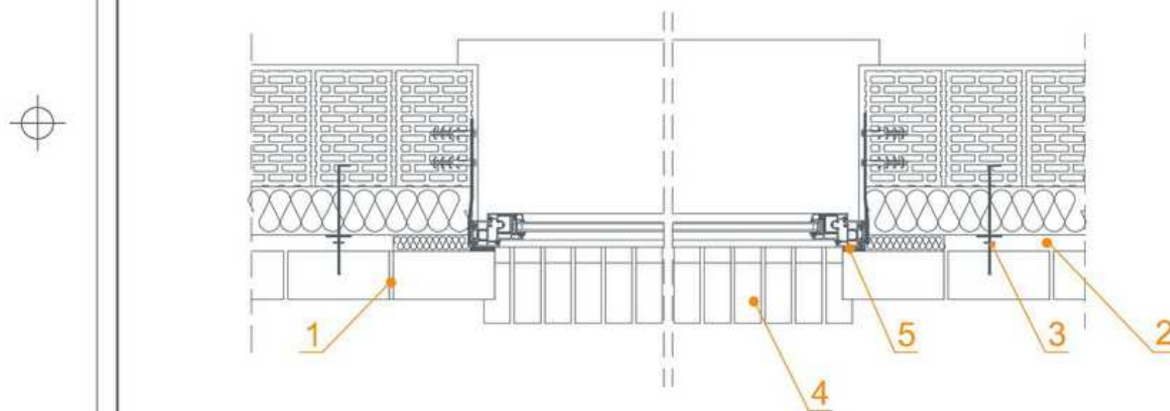
сечение A-A
