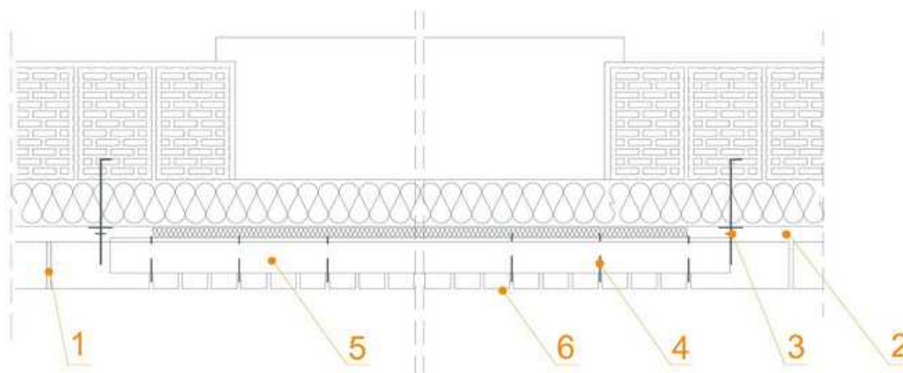
сечение A-A
