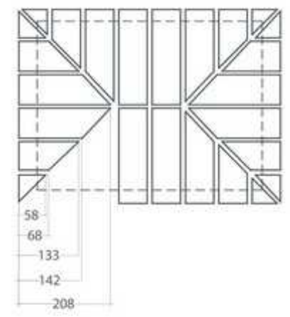
Форма OW1
