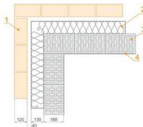
MAX 288x188x188/220, клинкерный кирпич 120 мм
