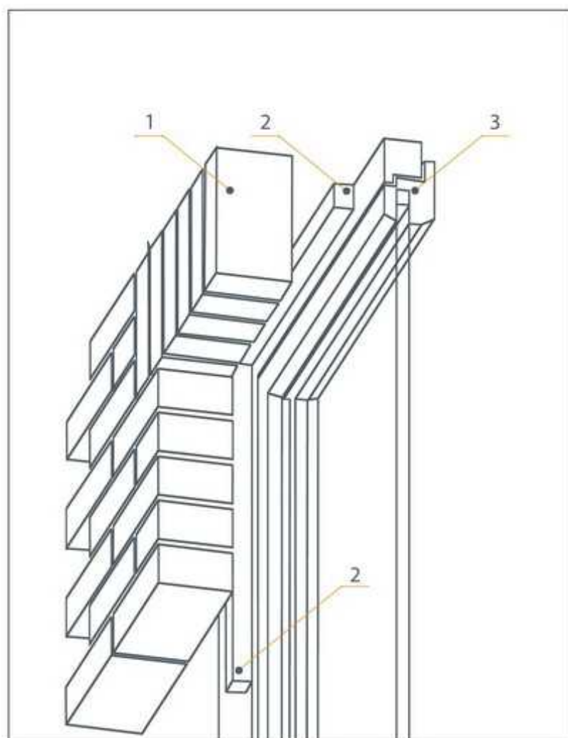
1 - кирпич клинкерный, 2 - демпферная лента, 3 - оконная коробка
