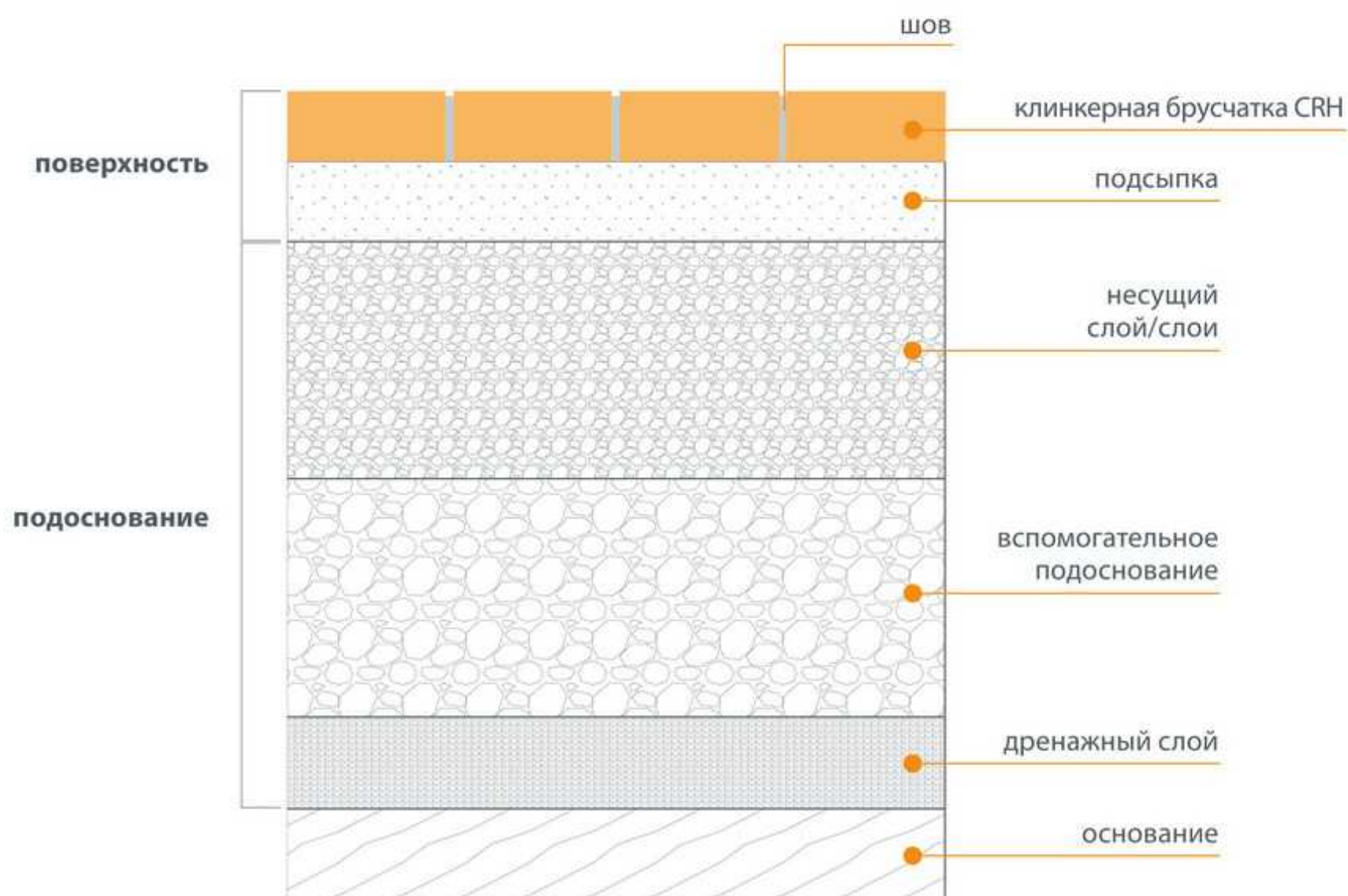
Сечение конструкции дороги.
