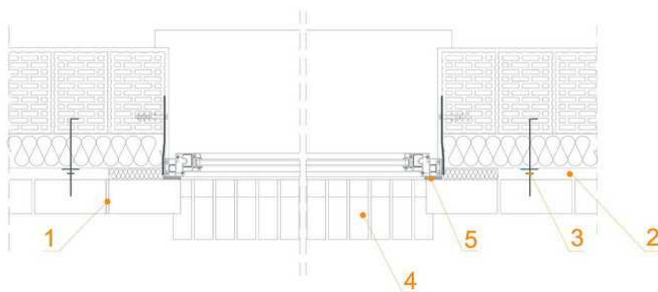
сечение А-А
