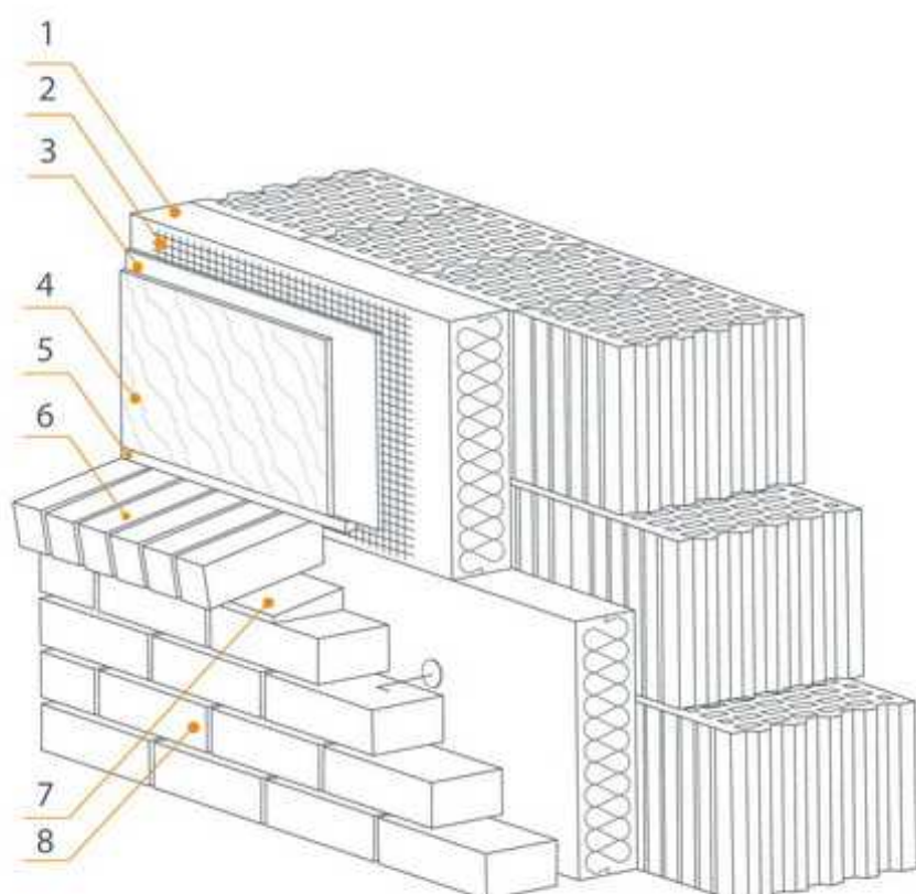
1 - термоизоляция, 2 - акриловая сетка, 3 - клей, 4 - штукатурка, 5 - уплотнительная лента, 6 - кирпич половинка, 7 - раствор, 8 - клинкерный кирпич
