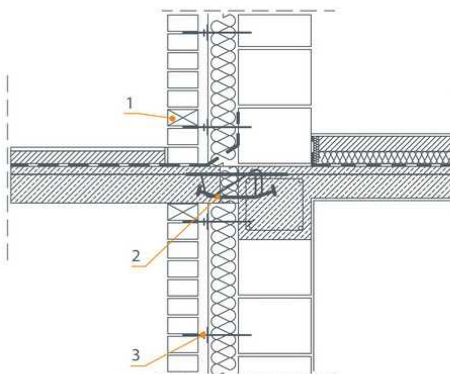
1 - коробка вентиляционная, 2 - балконный термосоединитель 3 - анкер
