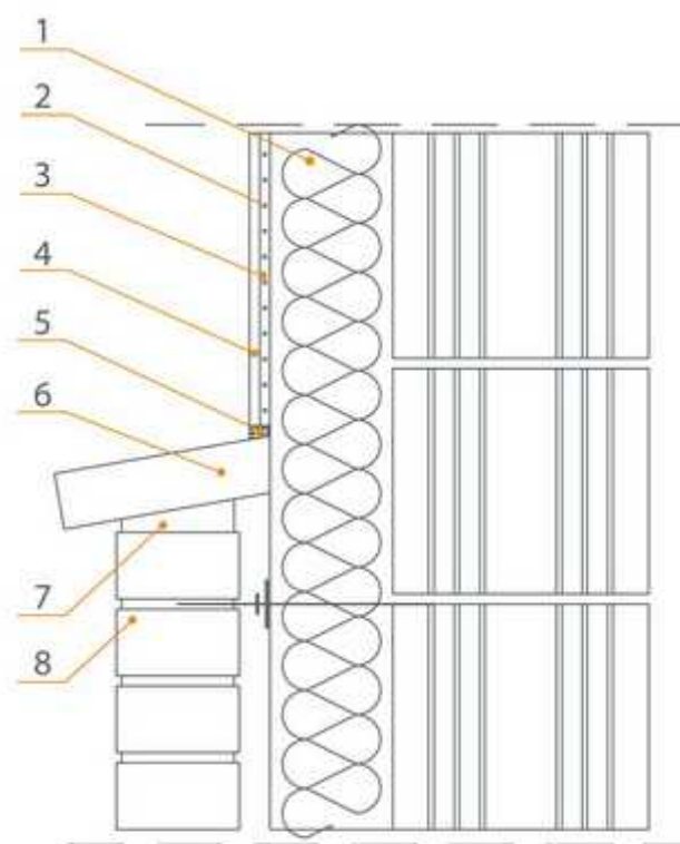
1 - термоизоляция, 2 - акриловая сетка, 3 - клей, 4 - штукатурка, 5 - уплотнительная лента, 6 - кирпич половинка, 7 - раствор, 8 - клинкерный кирпич
