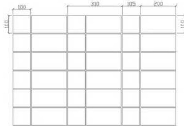
горизонтальный разрез
