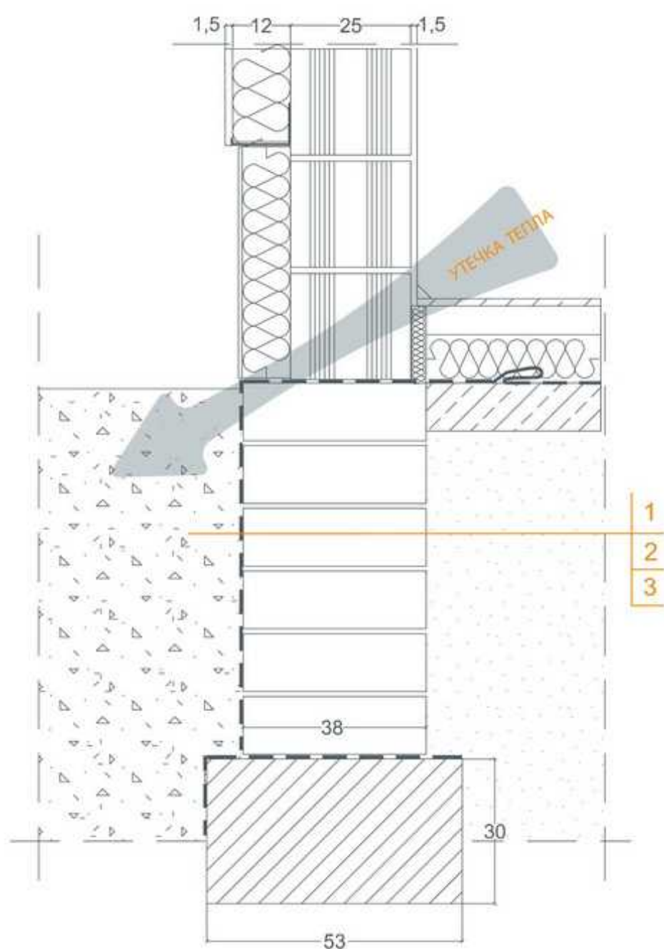
1 пленка, 2 гидроизоляция, 3 блоки бетонные 38x25x12 см
