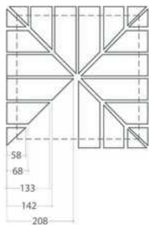
Форма P1
