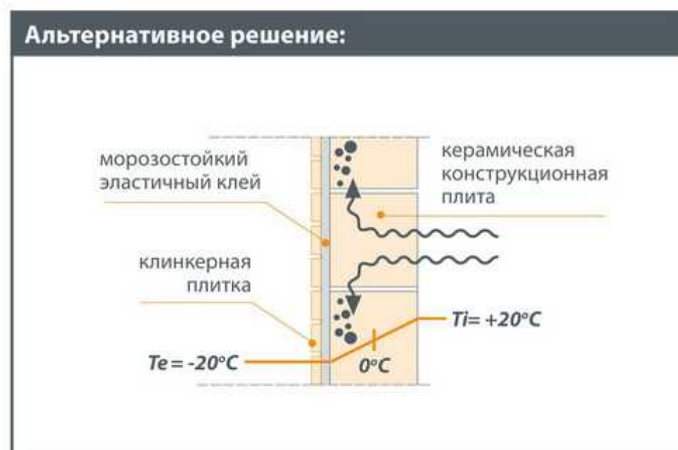
Распределение влажности и температур в однослойных стенах вентилируемых и невентилируемых
