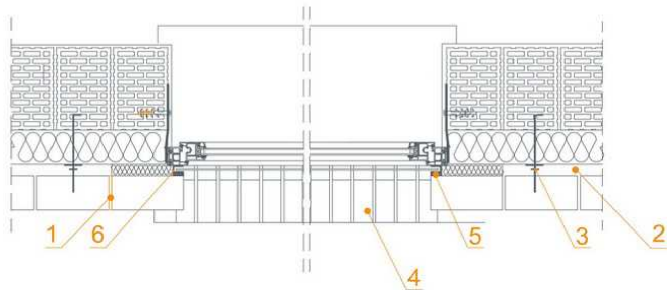
сечение A-A
