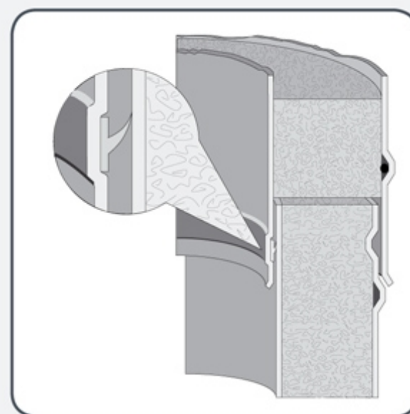
Соединение при избыточном давлении
