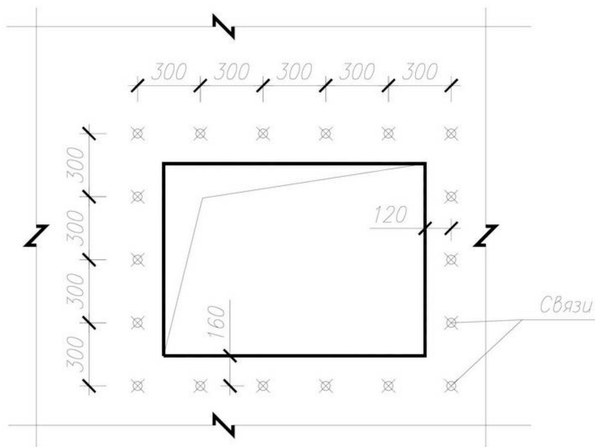
Рис.1 Схема установки связей у проемов.
