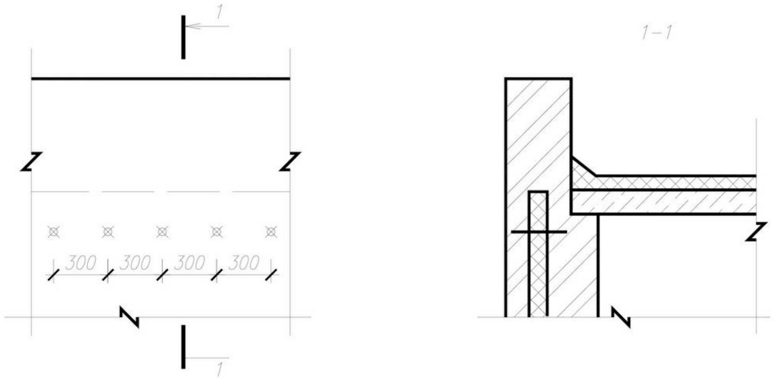
Рис.3 Схема установки связей у парапета.
