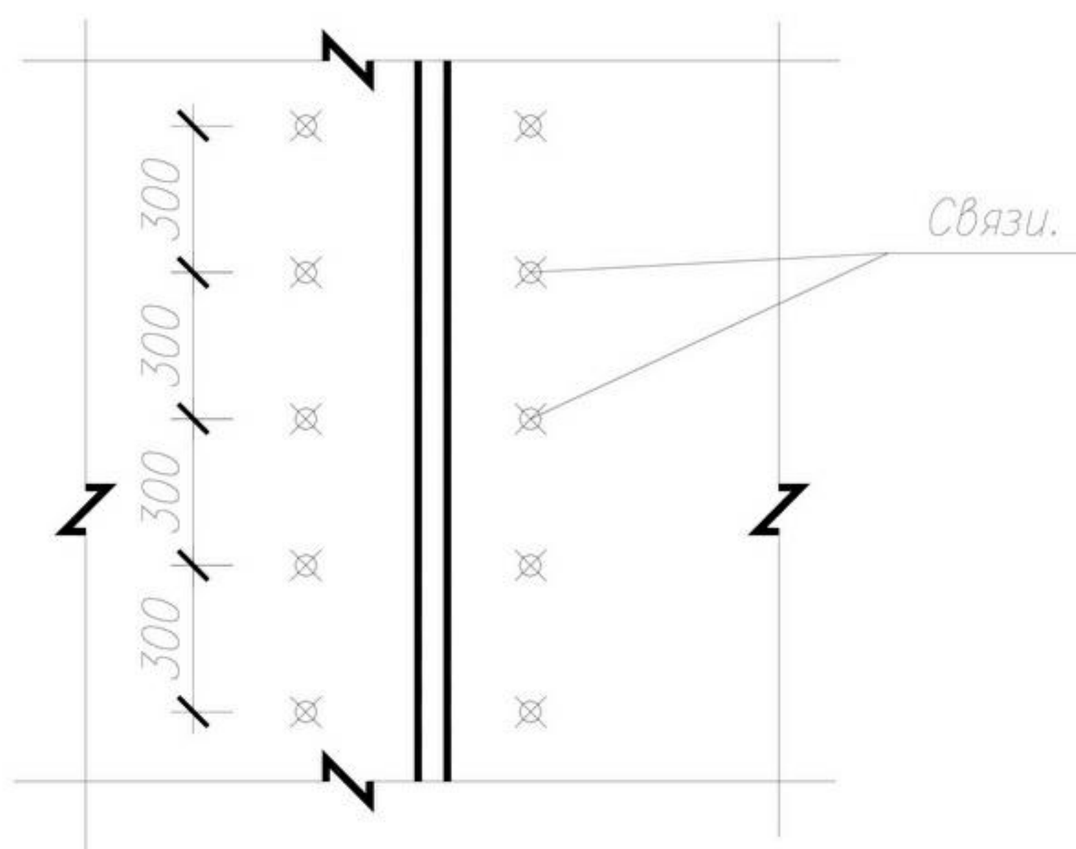
Рис.2 Схема установки связей у деформационного шва.
